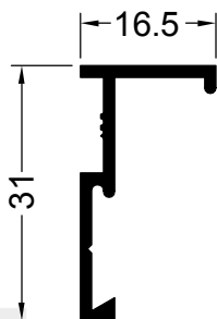
17038 0.211 Kg/m
