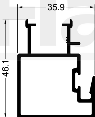
99054 0.700 Kg/m
