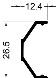
12549 0.132 Kg/m
