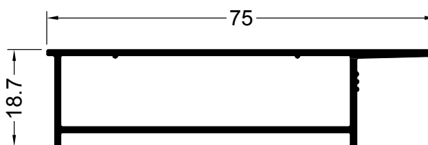
12662 0.563 Kg/m
