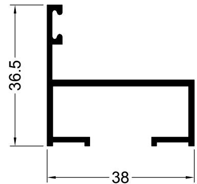
10670 0.453 Kg/m MAX-AIR MARCO 38 mm.
