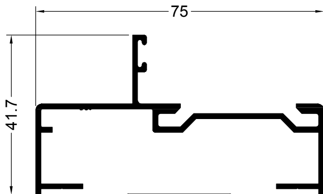
11253 0.715 Kg/m PUERTA MARCO ENCOLIZADO
