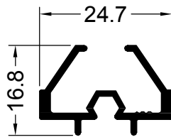
12249 0.232 Kg/m
