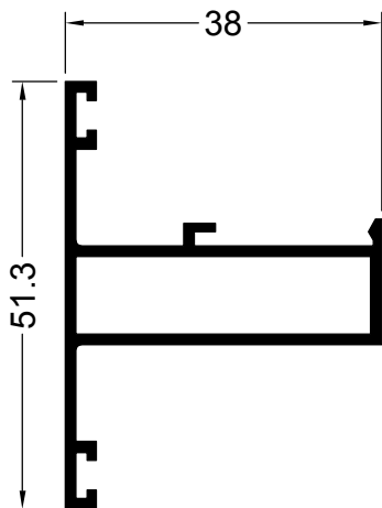
10741 0.543 Kg/m MAX-AIR HOJA APERTURA EXTERIOR
