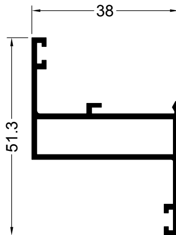
10669 0.543 Kg/m MAX-AIR HOJA 38 mm.
