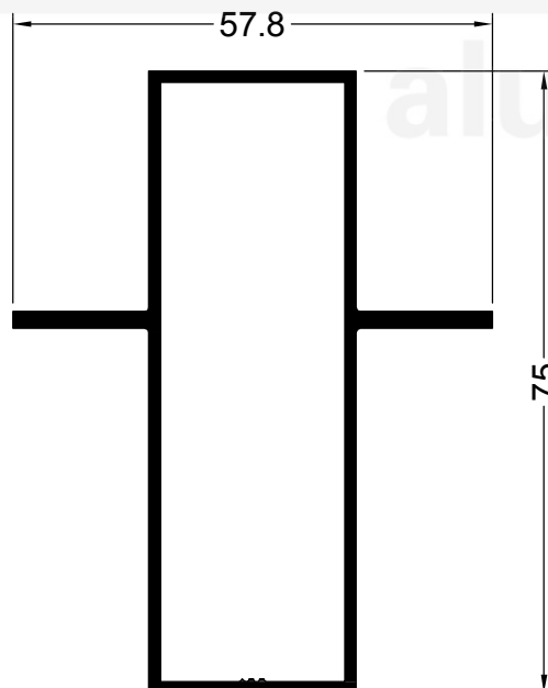
17034 0.915 Kg/m
