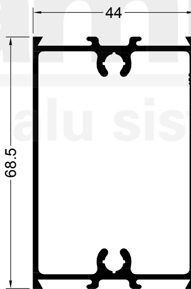
11256 1.040 Kg/m PUERTA HOJA UMBRAL/DINTEL/TRAVESAÑO
