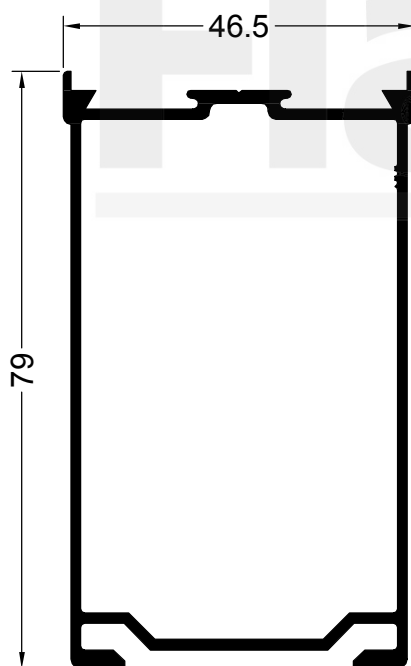
11252 1.015 Kg/m PUERTA HOJA ENCOLIZADA
