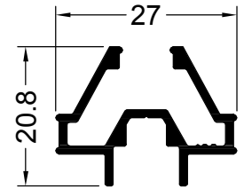
11198 0.293 Kg/m
