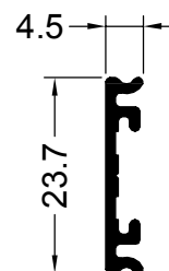
12550 0.138 Kg/m
