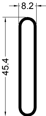
10992 0.300 Kg/m POSTIGON TABLILLA TUBULAR
