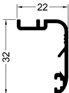
12540 0.281 Kg/m
