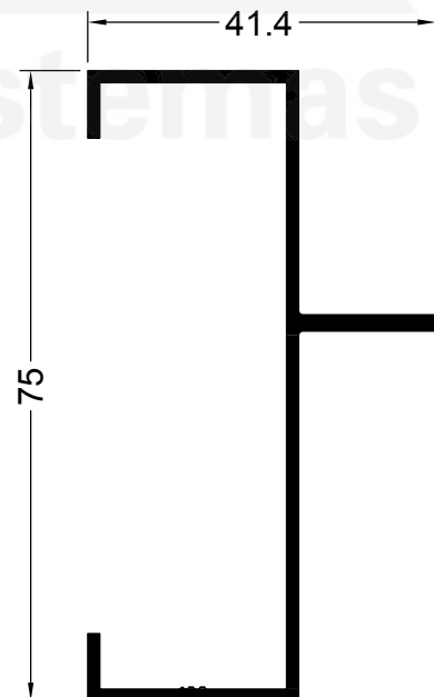
17035 0.603 Kg/m
