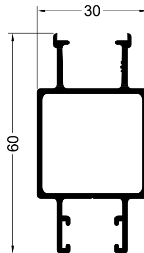
99053 0.712 Kg/m
