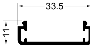
11867 0.227 Kg/m POSTIGON SOPORTE TABLILLA 10992
