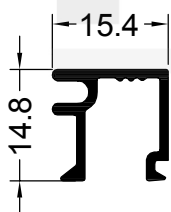
99008 0.165 Kg/m
