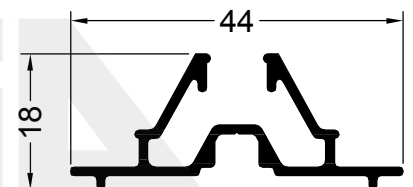
11874 0.335 Kg/m
