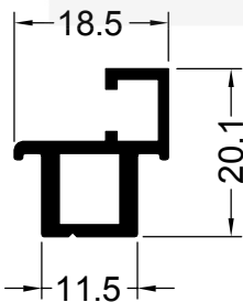
13332 0.273 Kg/m MOSQUITERO POSTIZO
