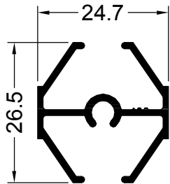
12232 0.309 Kg/m
