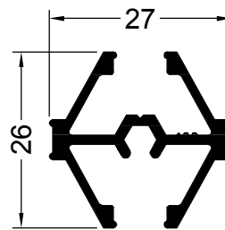
11197 0.386 Kg/m
