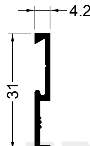
17039 0.160 Kg/m
