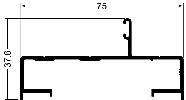
11101 0.676 Kg/m PUERTA MARCO SIN ENCOLIZAR
