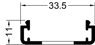
11978 0.190 Kg/m POSTIGON SOPORTE TABLILLA 10992 MECANIZADO
