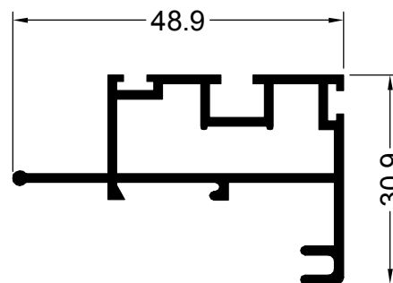
11156 0.589 Kg/m GUILLOTINA HOJA UMBRAL/DINTEL
