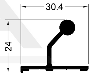
12189 0.315 Kg/m VENTILUZ HOJA BISAGRA
