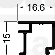
17006 0.170 Kg/m
