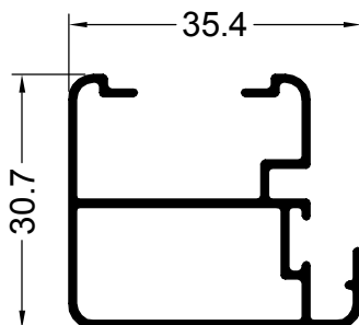
12585 0.401 Kg/m
