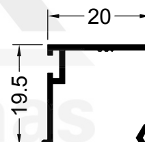
10744 0.171 Kg/m
