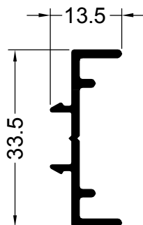
12705 0.248 Kg/m
