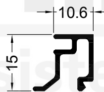
11746 0.157 Kg/m
