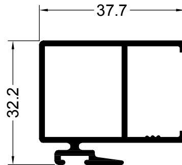
99250 0.573 Kg/m CORREDIZA HOJA ENCUENTRO DVH
