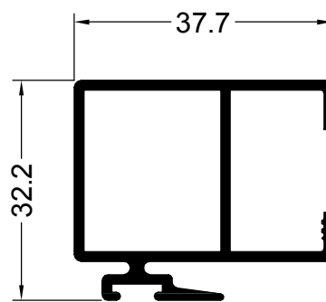
99207 0.605 Kg/m CORREDIZA HOJA ENCUENTRO V. SIMPLE
