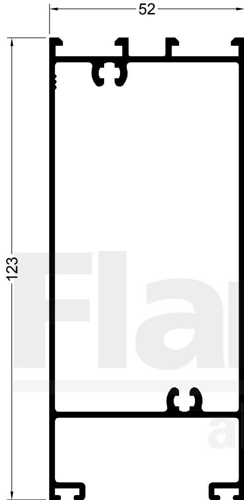
99319 1.660 Kg/m PUERTA HOJA ZOCALO
