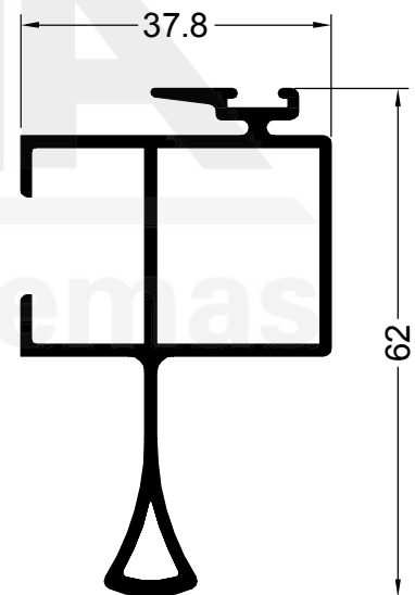
99208 0.813 Kg/m CORREDIZA HOJA ENCUENTRO C/ASA V. SIMPLE
