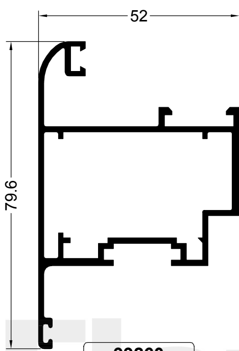
99260 1.120 Kg/m DESPLAZABLE HOJA CURVA
