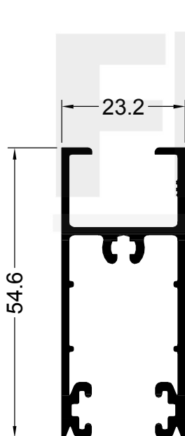
99204 0.667 Kg/m CORREDIZA HOJA DINTEL V. SIMPLE
