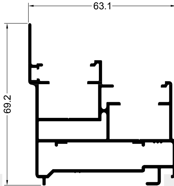
13153 1.225 Kg/m GUILLOTINA MARCO
