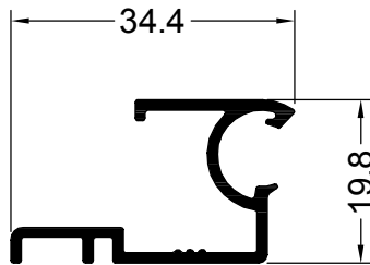
13904 0.298 Kg/m CORTINA BISAGRA MARCO PARA 13905
