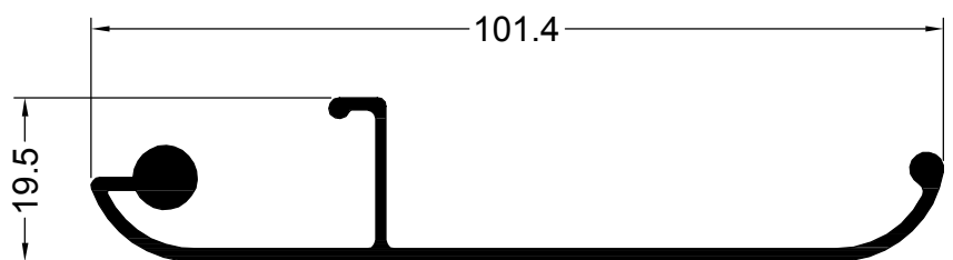
11651 0.695 Kg/m
