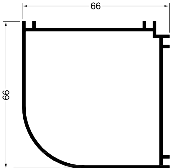
12512 0.978 Kg/m ACOPLE 90°
