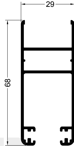
12699 0.855 Kg/m CORREDIZA HOJA DVH
