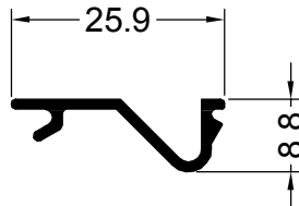
13154 0.138 Kg/m GUILLOTINA TAPA COMPENSADOR
