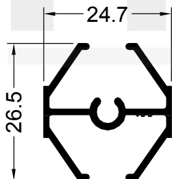
12232 0.309 Kg/m
