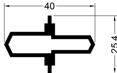
12650 0.481 Kg/m CORREDIZA ENCUENTRO 4 HOJAS
