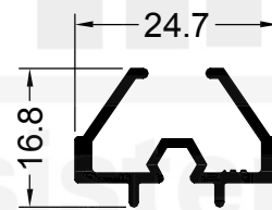
12249 0.232 Kg/m
