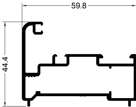
12510 0.877 Kg/m
