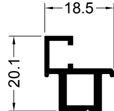
13332 0.273 Kg/m
