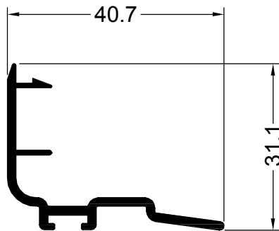
12700 0.356 Kg/m CORREDIZA HOJA ENCUENTRO
