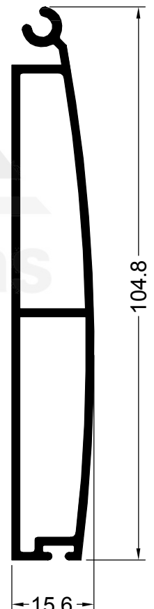
13462 1.002 Kg/m CORTINA ZOCALO
