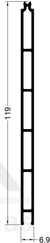
11781 0.894 Kg/m REVESTIMIENTO TUBULAR 119 mm.
