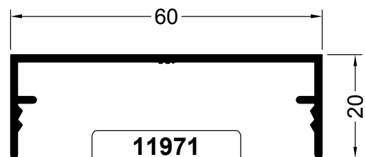
11972 0.461 Kg/m PRENSA VIDRIO
