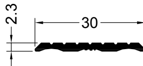
10981 0.144 Kg/m PUERTA TAPACANTO
