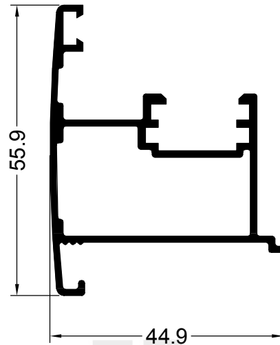
13170 0.729 Kg/m ABRIR ENCUESTRO 2 HOJAS
