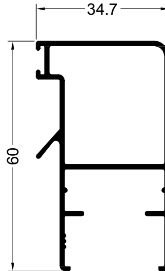
13335 0.670 Kg/m CORREDIZA HOJA ENCUENTRO DVH
