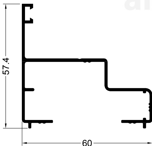
13561 0.645 Kg/m DESPLAZABLE MARCO
