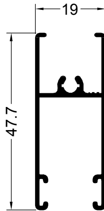
10812 0.393 Kg/m CORREDIZA HOJA DINTEL
