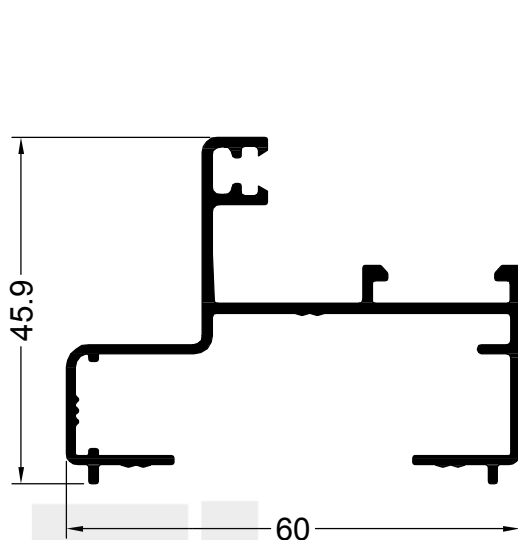
13172 0.656 Kg/m PAÑO FIJO/ABRIR MARCO
