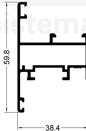
13223 0.707 Kg/m VENTILUZ HOJA
