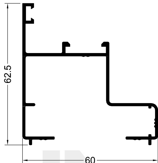
13247 0.732 Kg/m VENTILUZ MARCO
