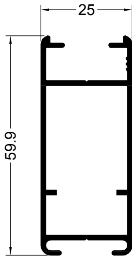
12204 0.668 Kg/m POSTIGON HOJA 60 mm.
