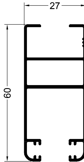
13237 0.657 Kg/m CORREDIZA HOJA JAMBA REFORZADA
