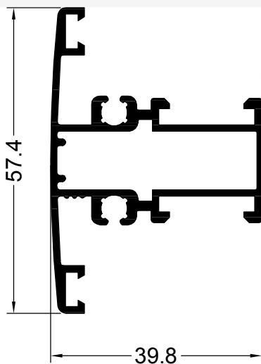
13173 0.794 Kg/m PAÑO FIJO/ABRIR TRAVESAÑO CURVO
