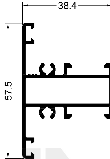
13230 0.750 Kg/m PAÑO FIJO/ABRIR TRAVESAÑO LIVIANO
