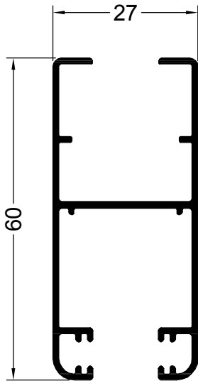
12919 0.595 Kg/m CORREDIZA HOJA JAMBA
