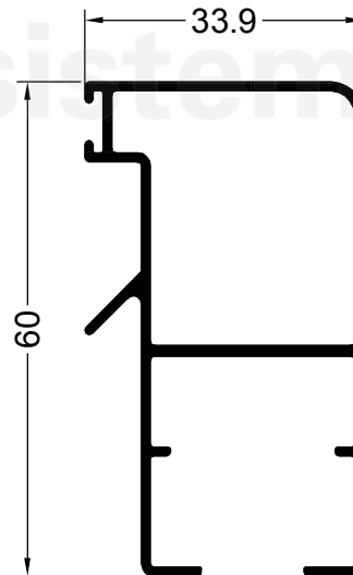
12932 0.639 Kg/m CORREDIZA HOJA ENCUENTRO
