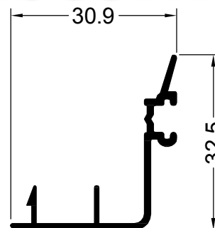
12581 0.258 Kg/m CORREDIZA HOJA ENCUENTRO
