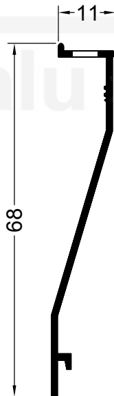
11199 0.272 Kg/m POSTIGON TABLILLA RECTA MECANIZADA
