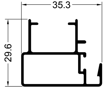
11961 0.375 Kg/m CORREDIZA HOJA ENCUENTRO
