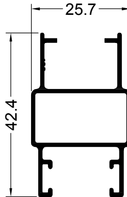
12706 0.398 Kg/m CORREDIZA HOJA JAMBA
