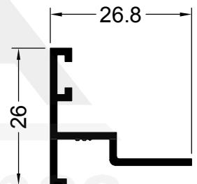
11632 0.223 Kg/m POSTIGON ENCUENTRO 2 HOJAS
