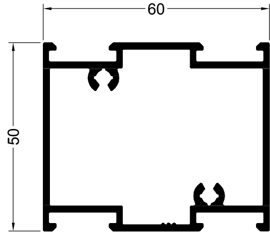
13661 1.260 Kg/m PUERTA TRAVESAÑO
