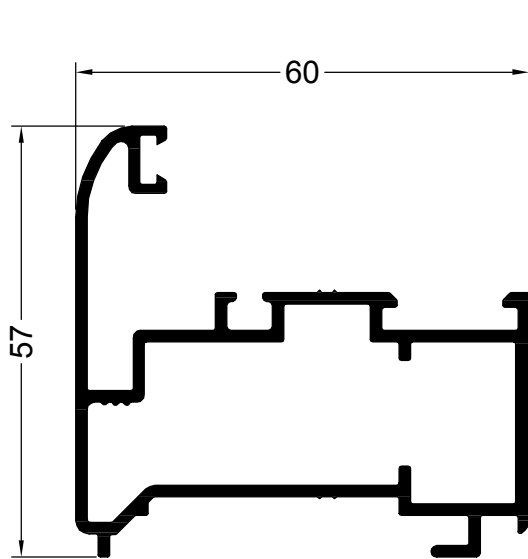
13162 1.116 Kg/m ABRIR/PAÑO FIJO MARCO
