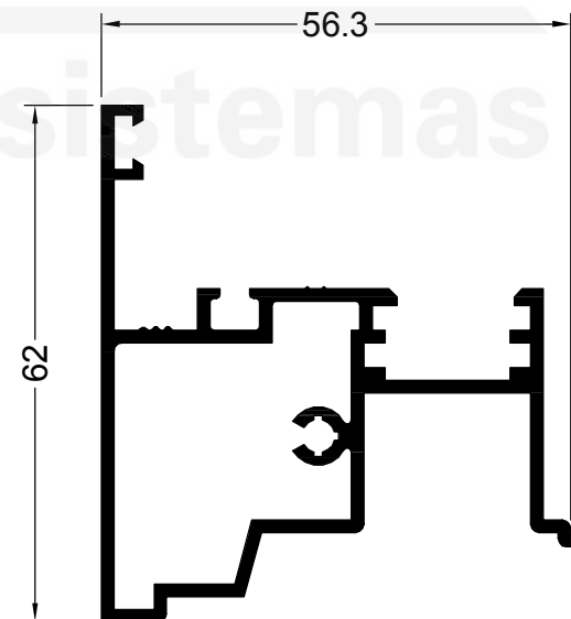
13164 1.062 Kg/m ABRIR ENCUENTRO 2 HOJAS
