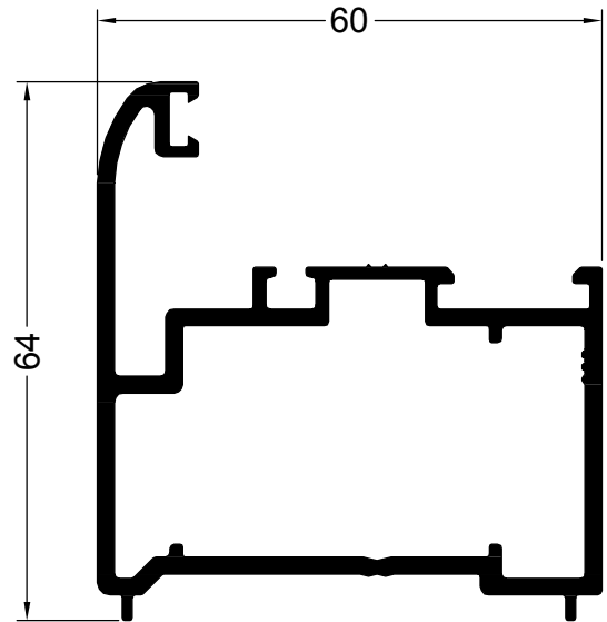
13746 1.394 Kg/m ABRIR/PAÑO FIJO MARCO REFORZADO
