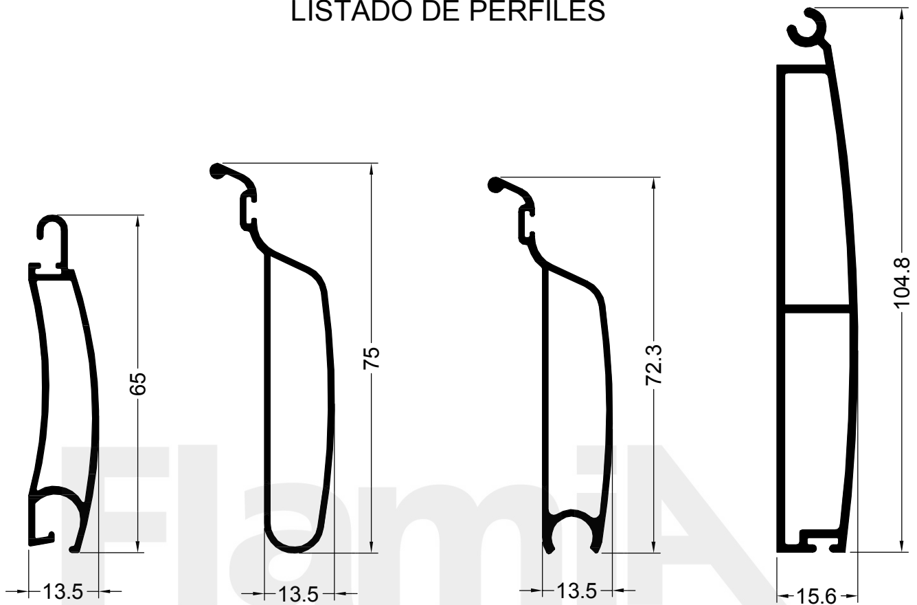
12646 0.499 Kg/m CORTINA TABLILLA CURVA
